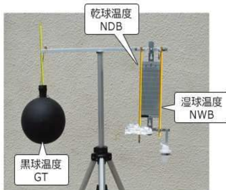
暑さ指数(WBGT)測定装置
